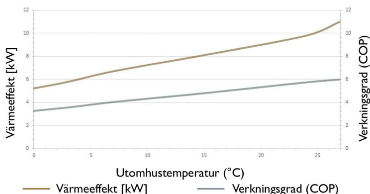
Värmeeffekt [kW] och verkningsgrad (COP) för V20 beroende på utomhustemperatur enligt NF 414
