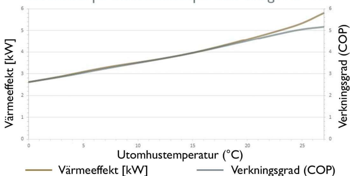
Värmeeffekt [kW] och verkningsgrad (COP) för P12 beroende på utomhustemperatur enligt NF 414
